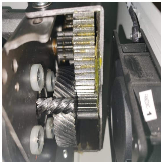
Engrenagem de tração em metal
